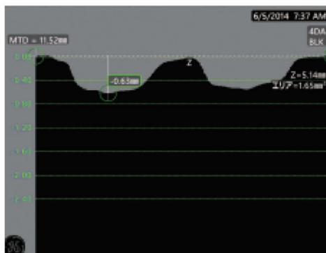
深さプロファイル
