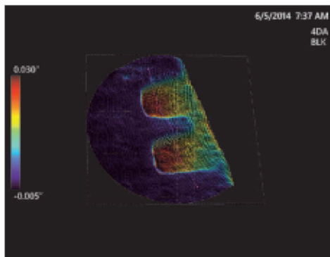
3D 点群画像
